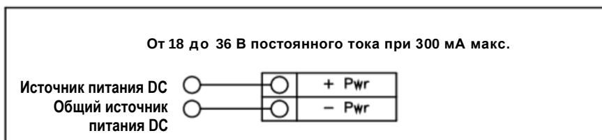
Рисунок 2-25. Подключение к источнику питания постоянного тока
