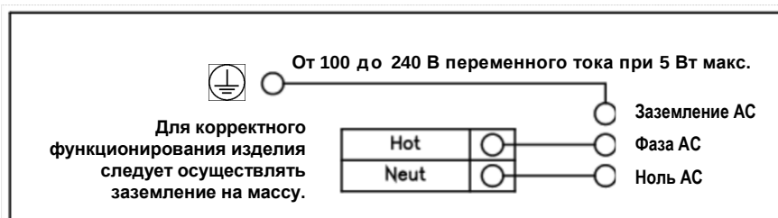
Рисунок 2-23. Подключение к источнику питания переменного тока
