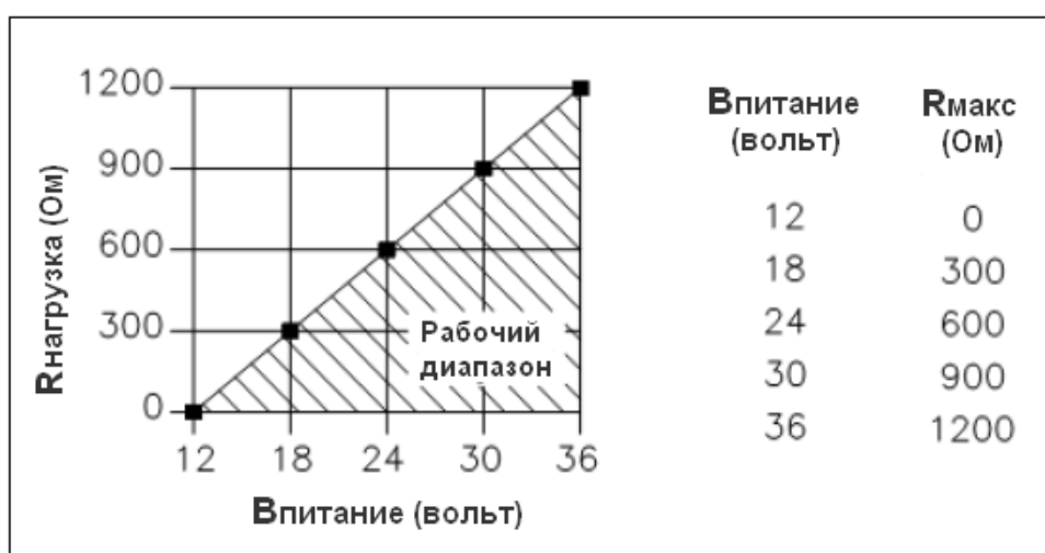
Рисунок 2-16. Зависимость сопротивления нагрузки от входного напряжения
