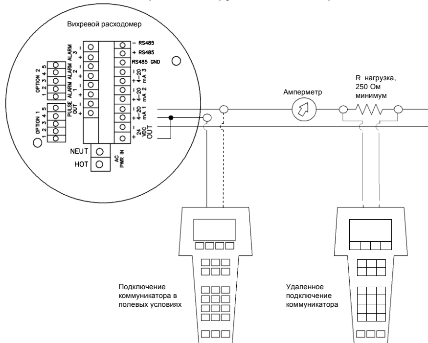
Рисунок 4-3. Подключение к расходомеру с питанием переменным током (HART)
