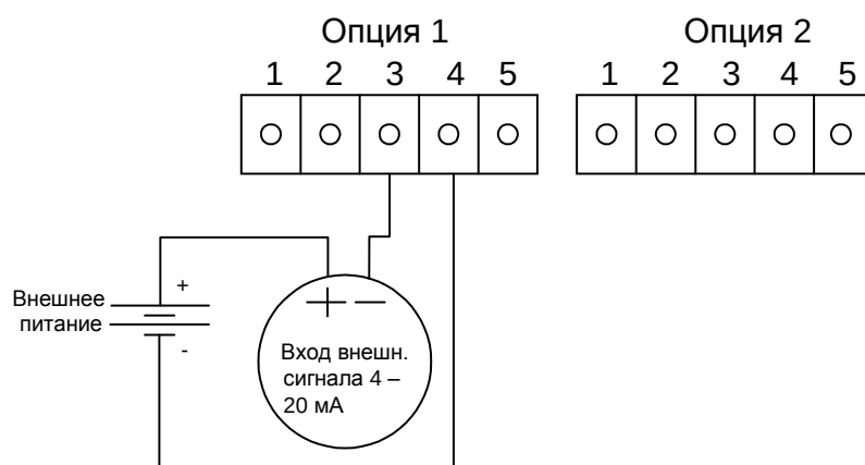
Рисунок 2-38. Подключение входа внешнего сигнала 4 – 20 мА – внешний источник питания
