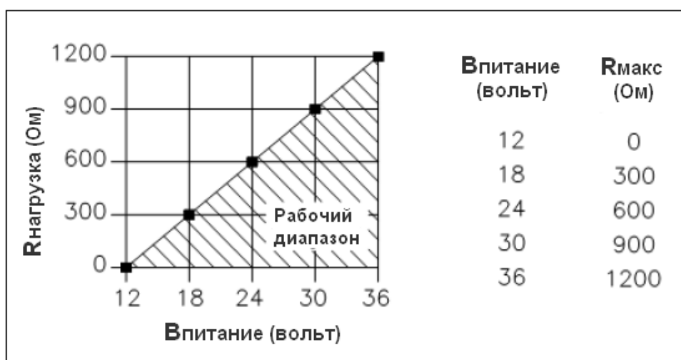
Рисунок 2-26. Зависимость сопротивления нагрузки от входного напряжения
