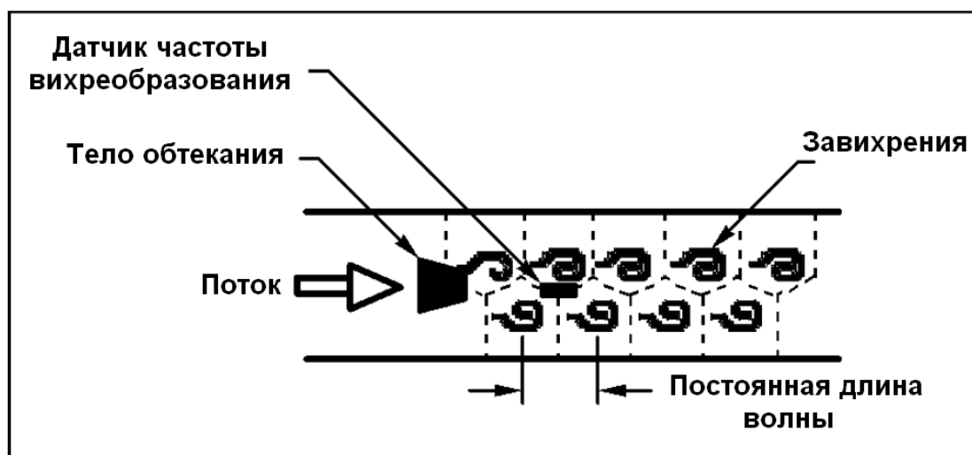
Рисунок 1-2. Принцип действия вихревых расходомеров
