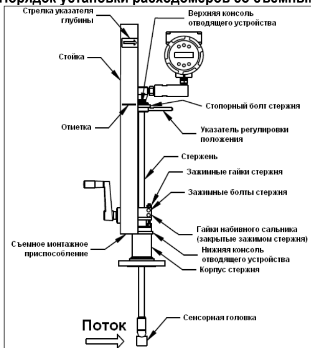
Рисунок 2-10. Расходомер со съемным монтажным приспособлением
