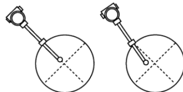
Правильная установка
