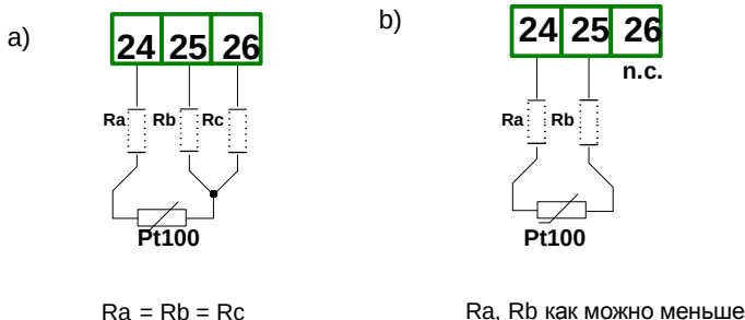
Рис. 4.9. Присоединение Pt100 датчика к каналу № 1:
