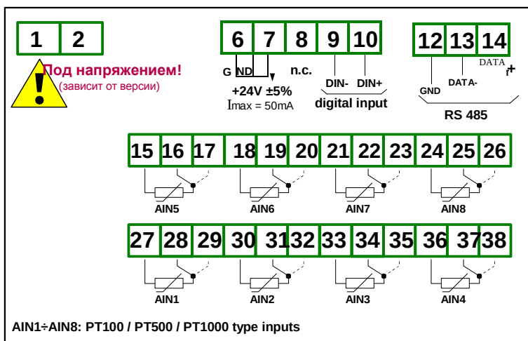
Fig. 4.6. Описание терминалов
